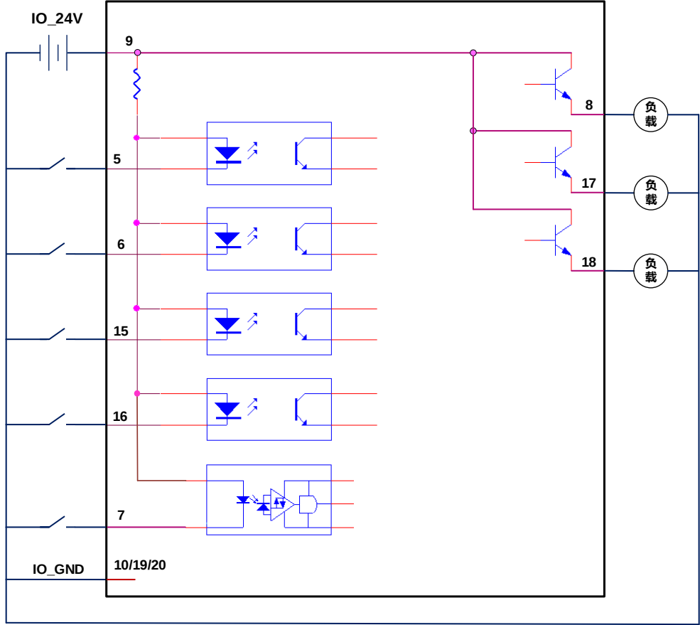
图 18 J08 的 IO 口接线说明
