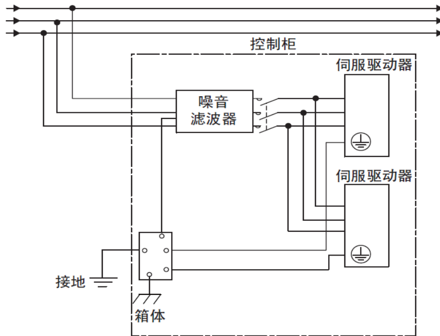
图 29 噪音滤波器接地线和控制柜内其他设备接线示意图
