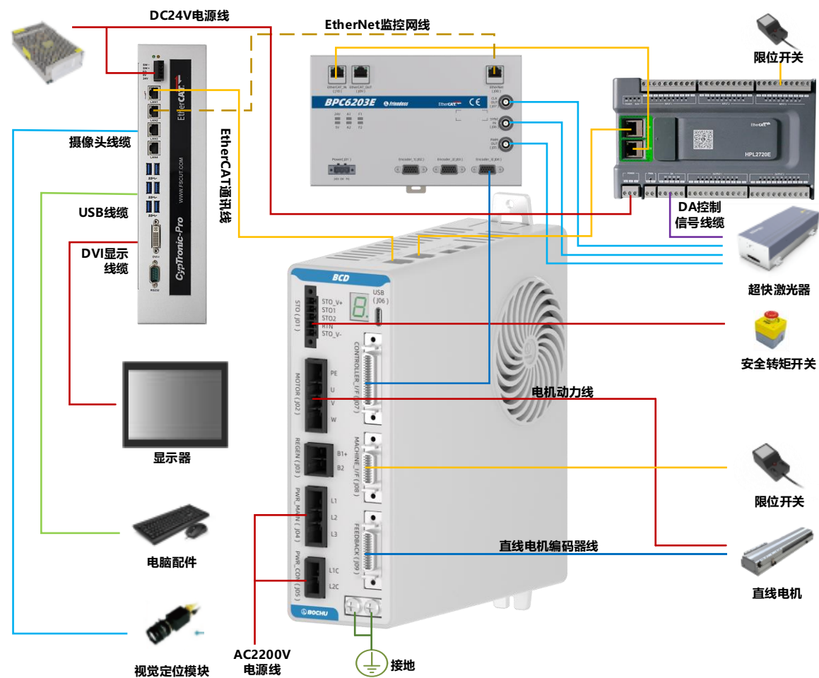
图 14 BCD113 驱动器配 7000S 系统的接线框图
