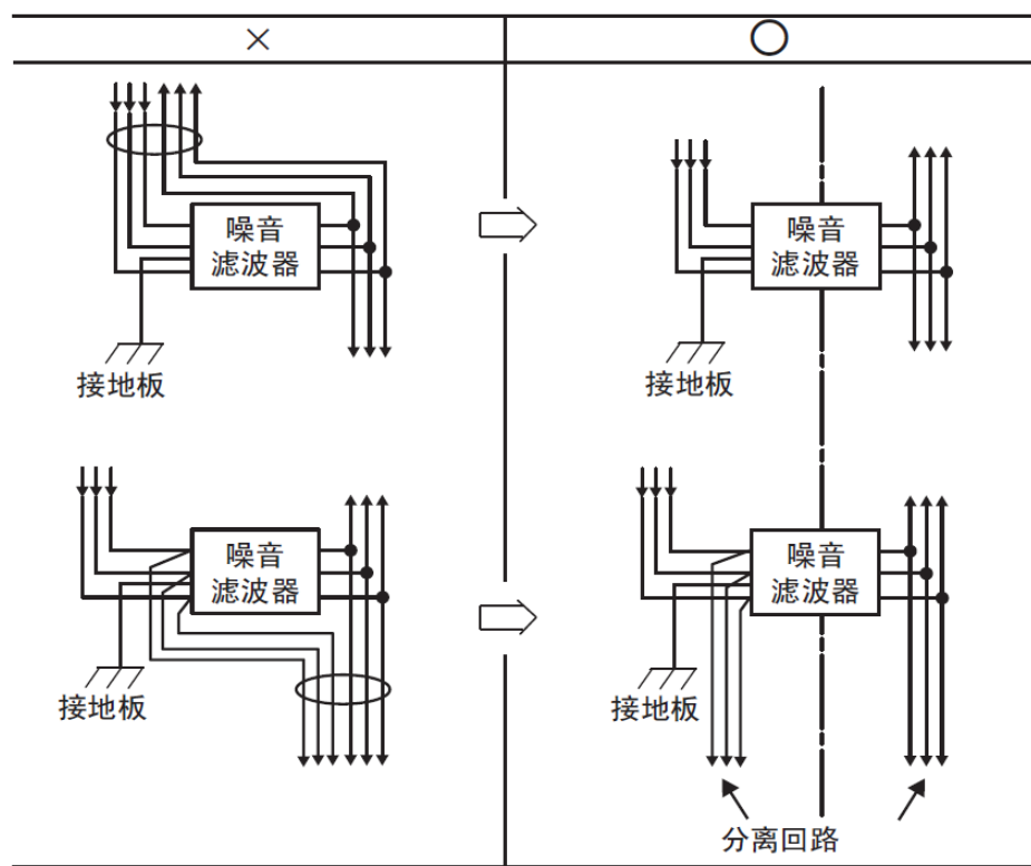
图 26 噪音滤波器输入接线与输出接线示意图
