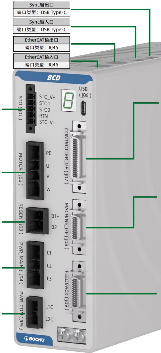
图 12 BCD113 的接口定义
