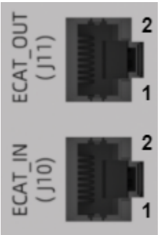
图 19 J10/J11 EtherCAT 通讯端子说明
