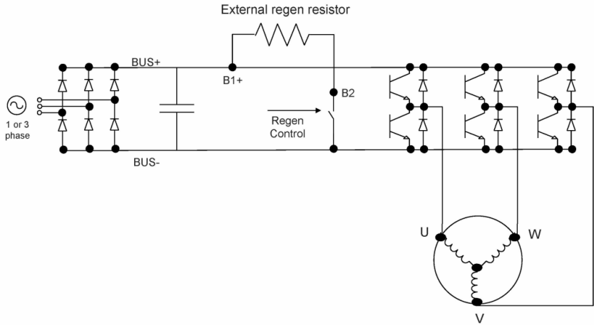
图 21 工作电路
