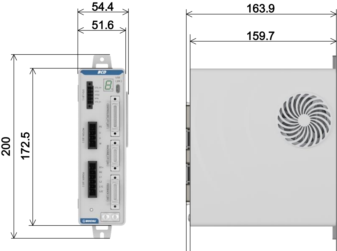
图 5 BCD105 尺寸
