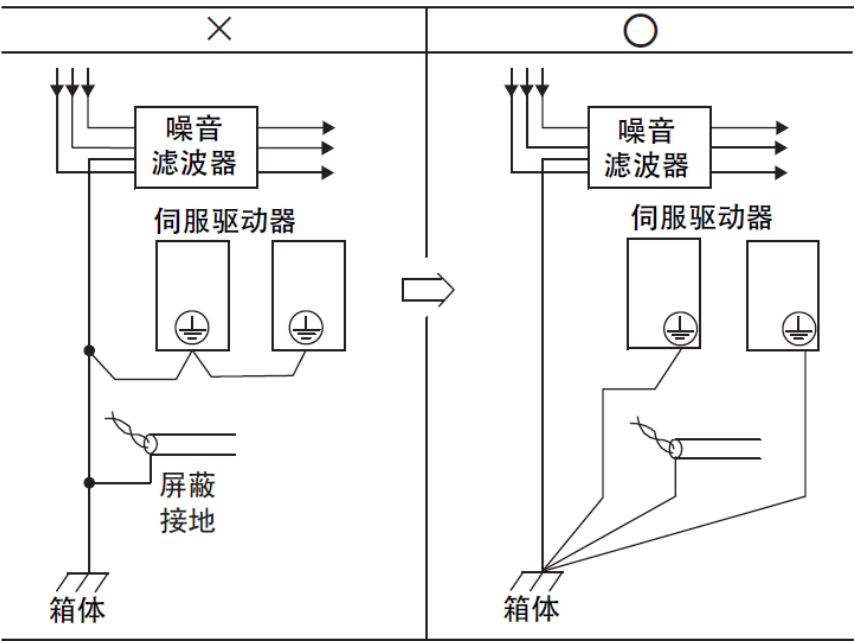
图 28 噪音滤波器接地线示意图
