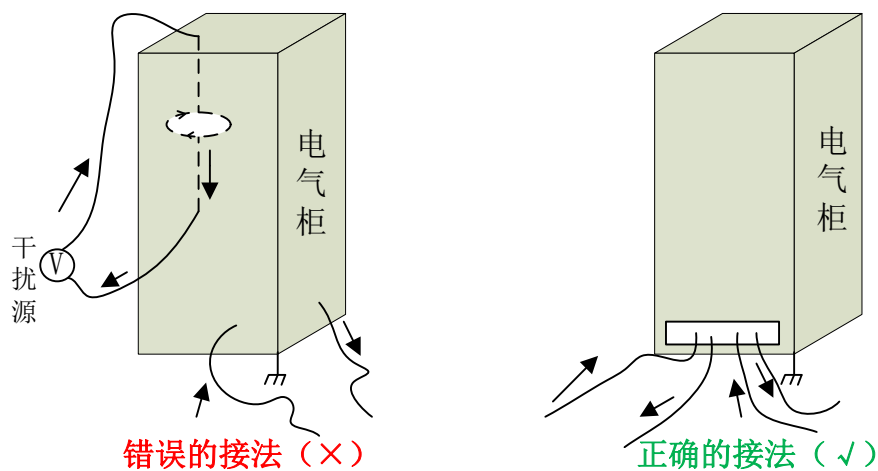
图 24 布线避免形成环路
