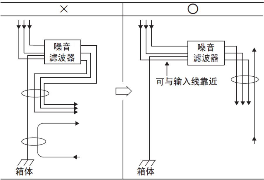
图 27 噪音滤波器接地线与输出接线示意图
