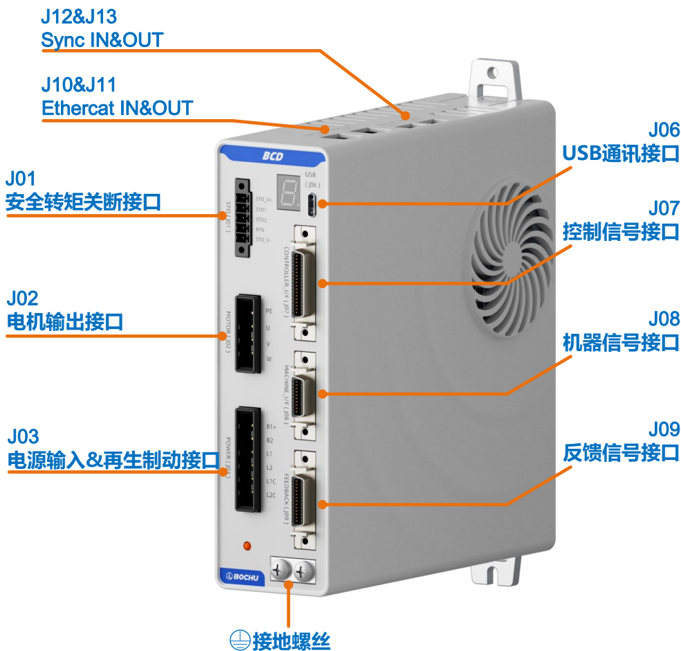
图 8 BCD105 的接口分布
