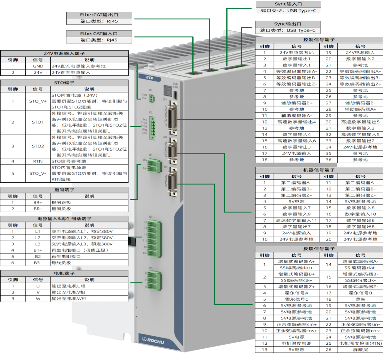
图 13 BCD125B 的接口定义
