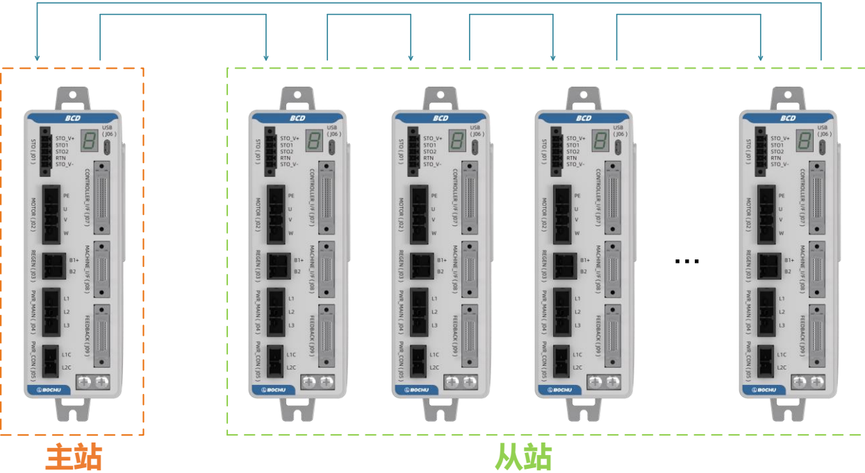
图 20 同步通讯接线图
