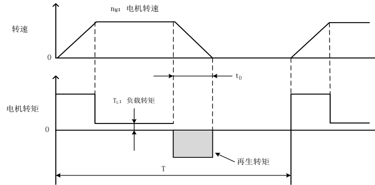
图 22 再生电阻器消耗能量图
