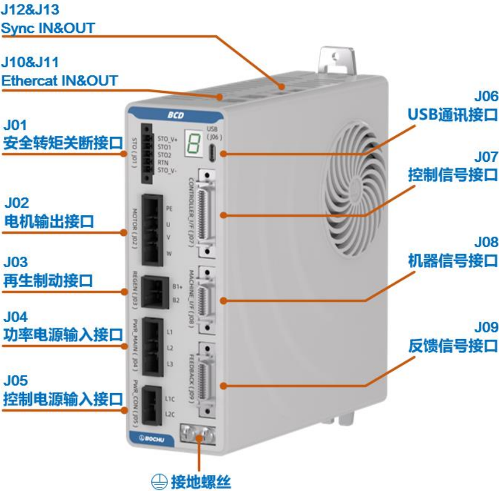
图 9 BCD113 的接口分布
