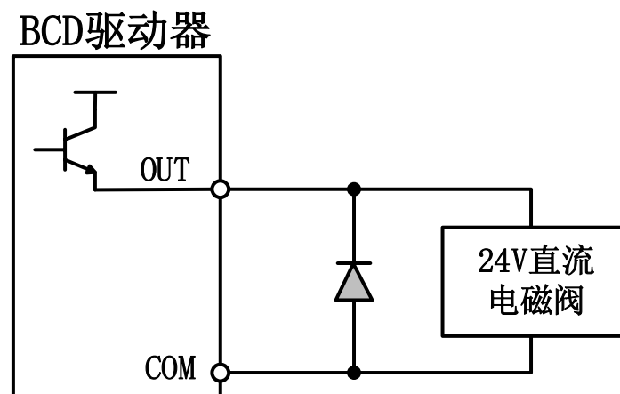
图23 电磁阀端加吸收电路图示
