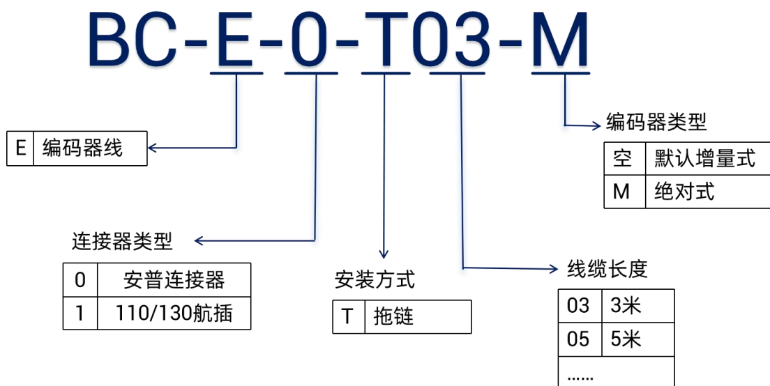
图 5 编码器线束型号说明
