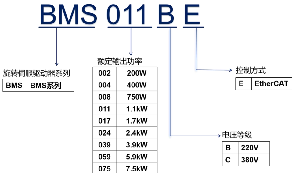
图 1 驱动器型号说明
