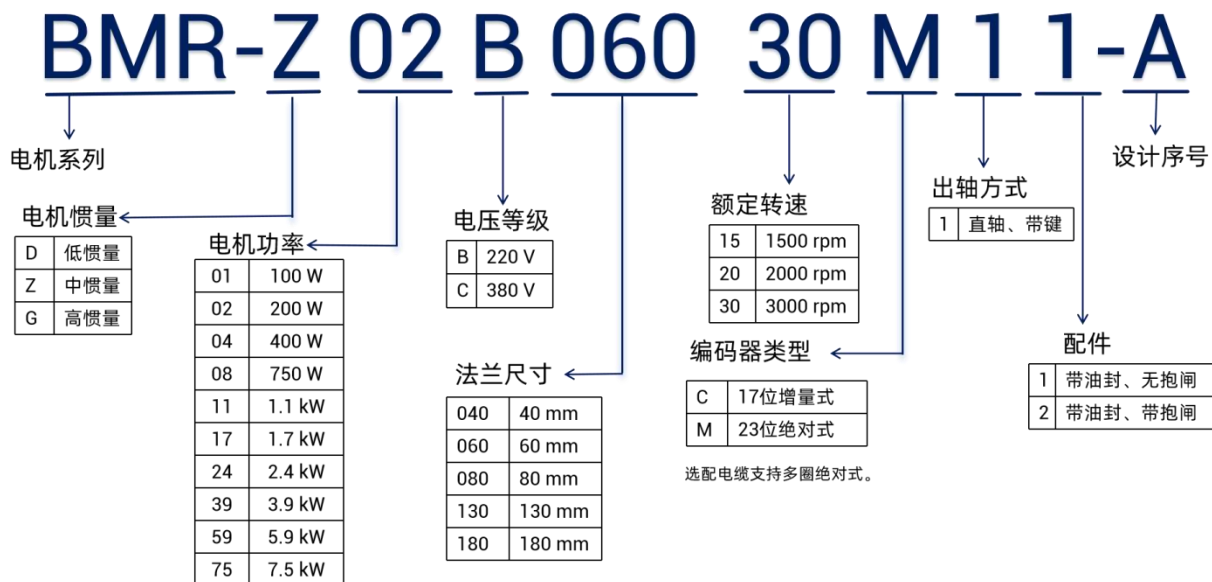
图 2 电机型号说明
