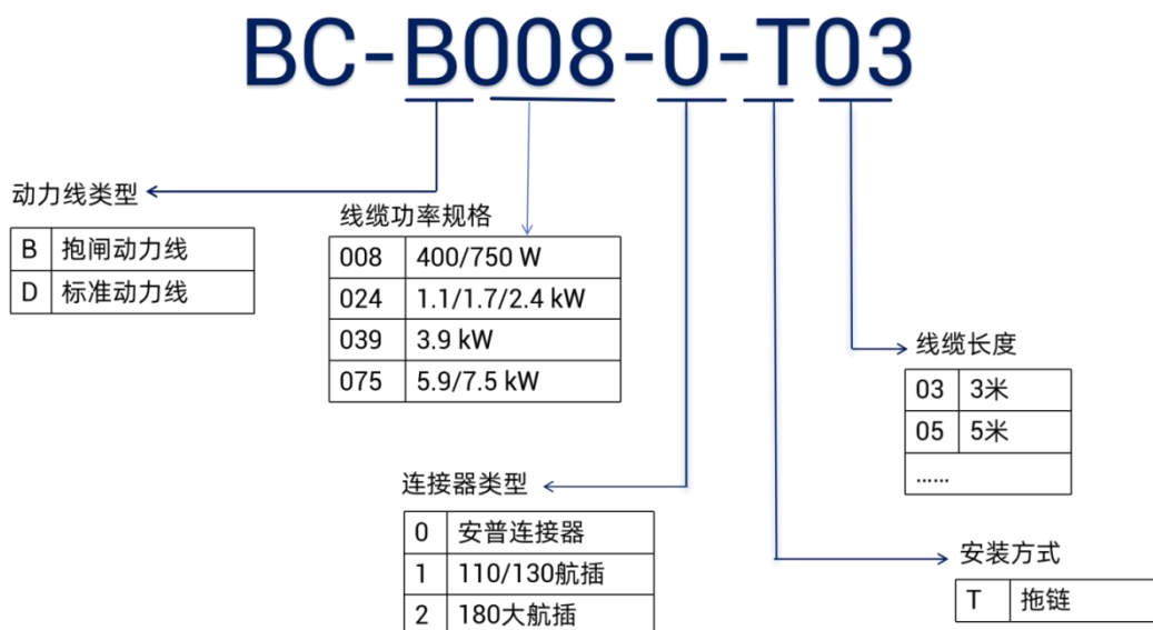
图 4 动力线束型号说明
