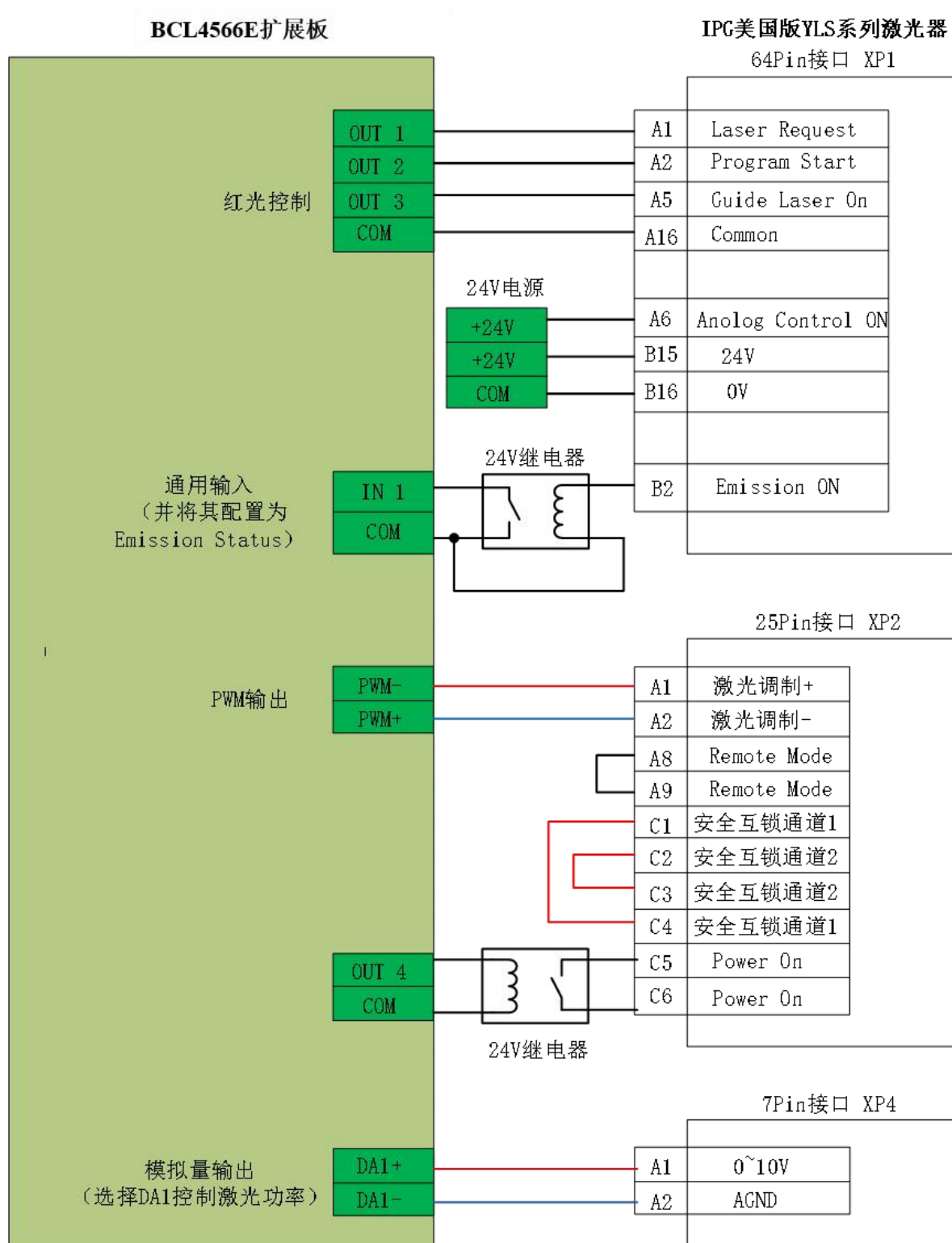
图 5-2 IPG-美国版非网络通讯接线图
