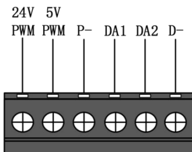
图 3-5 PWM/DA 接线端子
