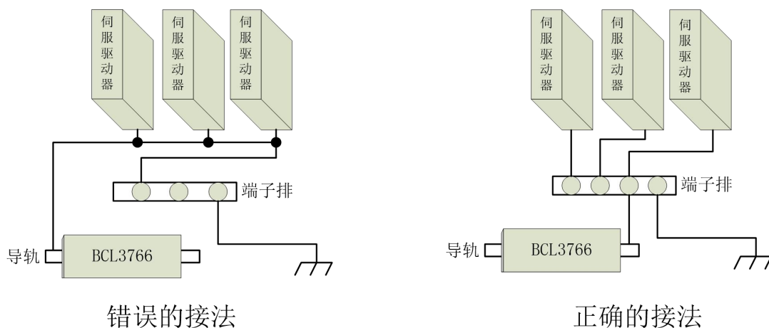
图 7-5 星形连接示意图
