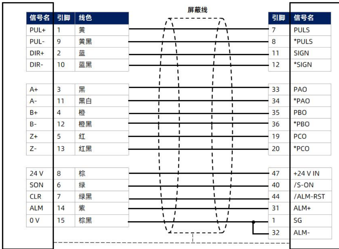
图 3-16 安川伺服接线图
