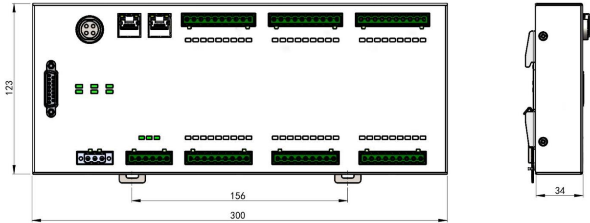
图 3-2 BCL4566E 尺寸图 (单位: mm)
