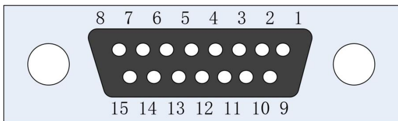
图 3-15 伺服驱动器接口说明
