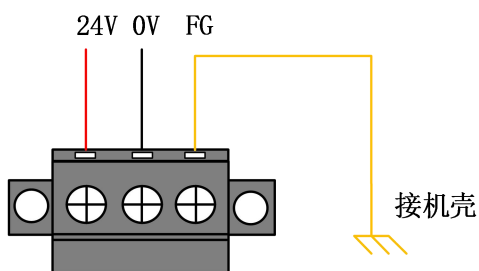
图 3-4 电源接口端子
