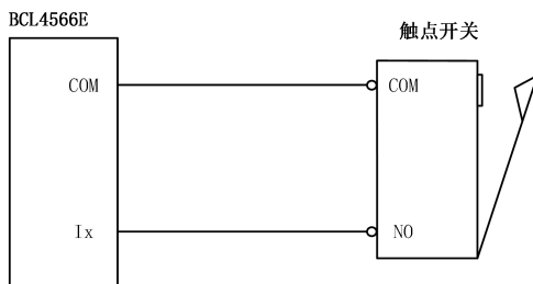
图 3-10 触点开关接线
