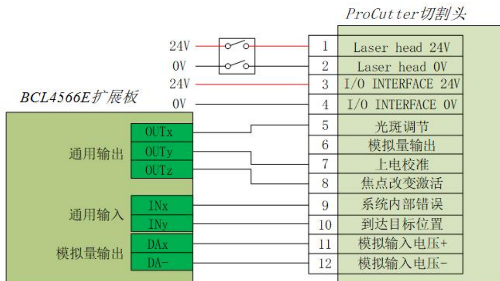
图 4-1 ProCutter 切割头连接
