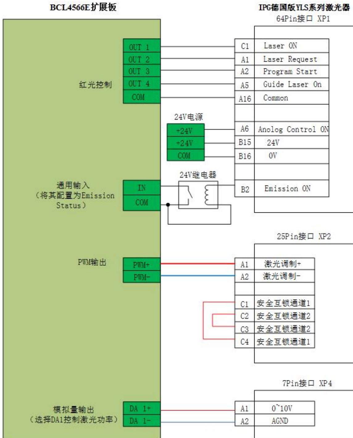
图 5-1 IPG-德国版非网络通讯接线图
