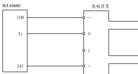
图 3-9 光电开关接线
