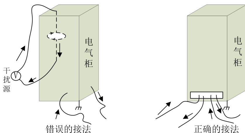
图 7-4 电气柜接线示意图
