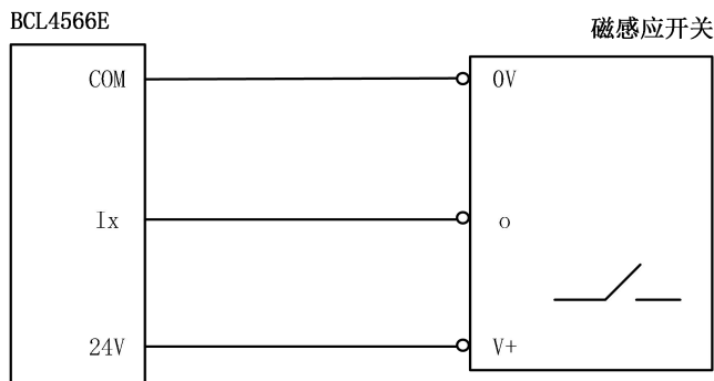
图 3-11 磁感应开关接线
