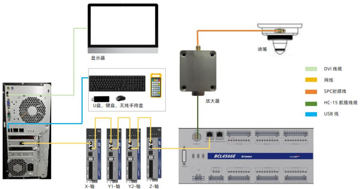
图 1-1 系统接线图
