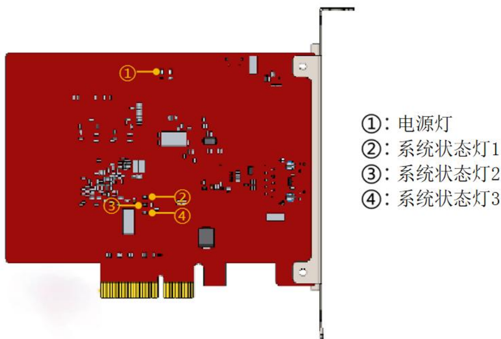
图 8-1 BMC228B 指示灯
