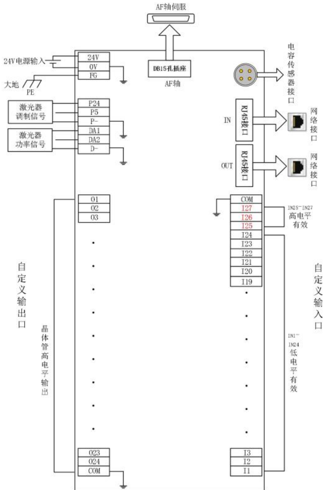
图 3-17 BCL4566E 接线图
