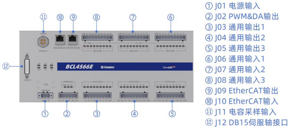
图 3-3 BCL4566E 接口布局
