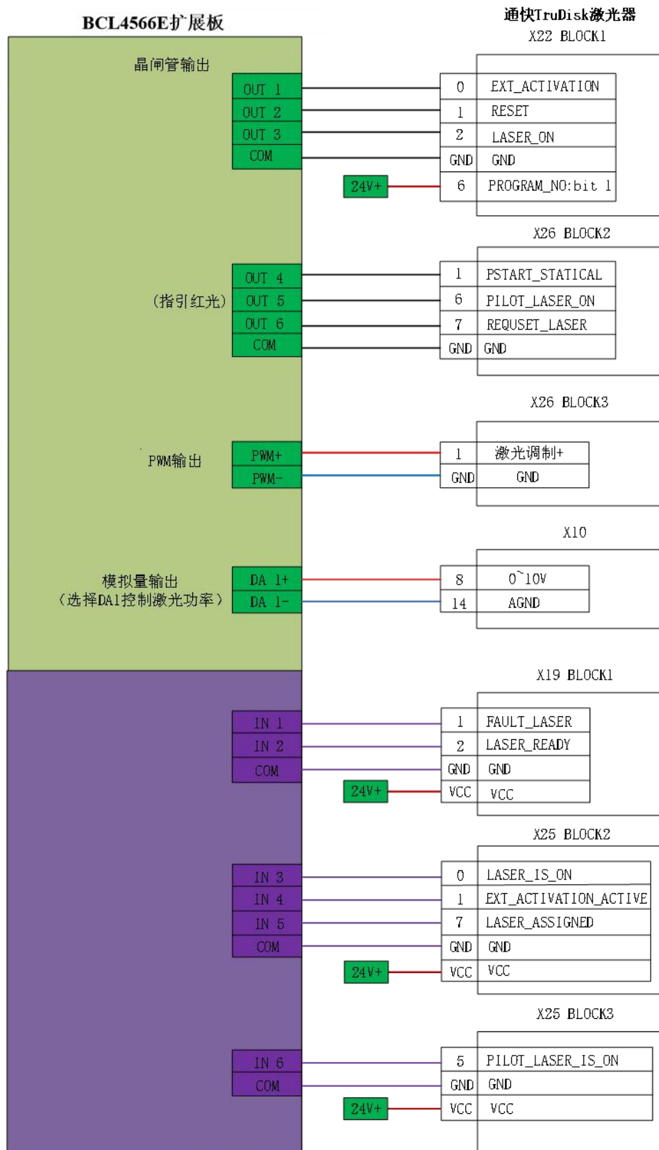
图 5-4 通快激光器接线图
