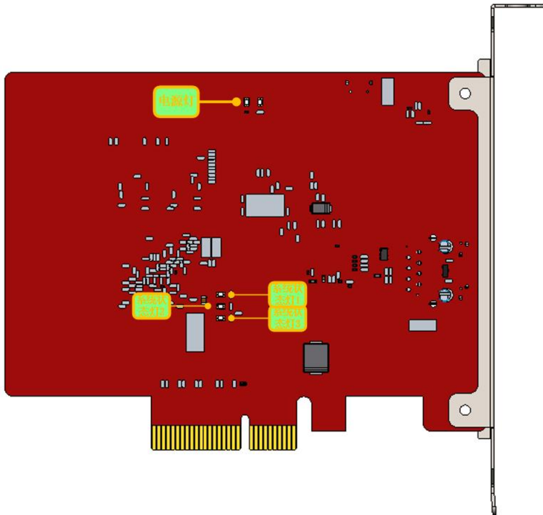
图 14 BMC228A 指示灯位置图
