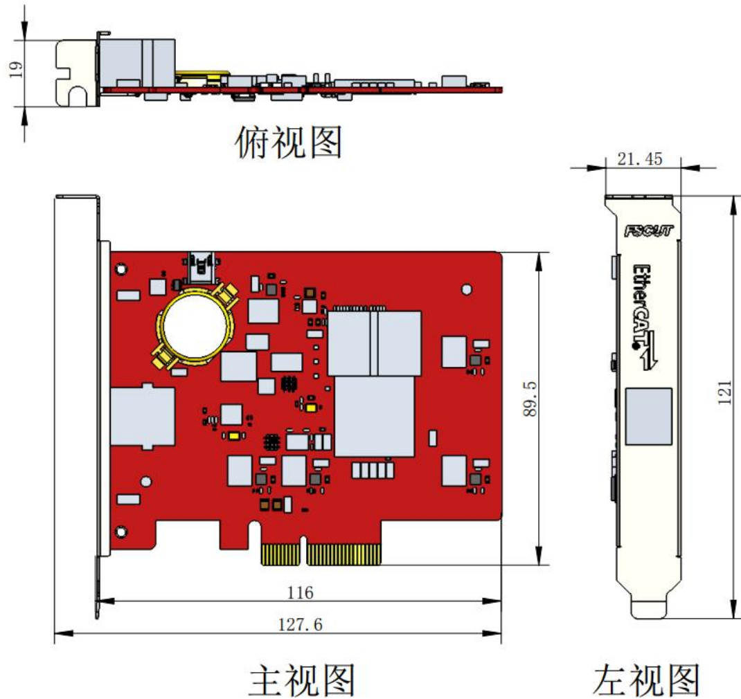
图 3 BMC228A 尺寸图
