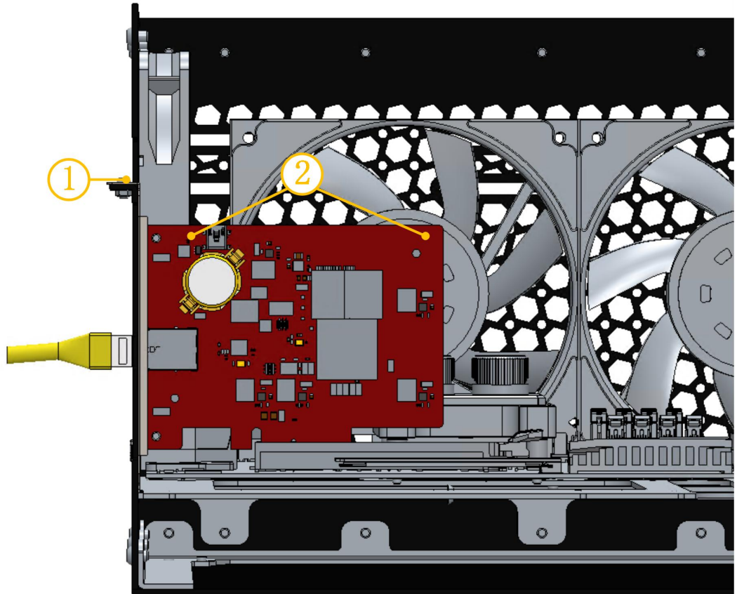
图 4 BMC228A 主站卡安装示意图
